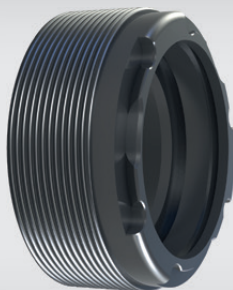
ERZD-Zeta Dichtspannmutter für Zollmann Dichtscheiben ERZD-Zeta seal nut for Zollmann sealing discs
