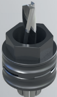
EDS-Zeta Eindrehhilfe zum manuellen Ansetzen der Spannmutter EDS-Zeta screw-on-adapter for manual placement of the collet nut on the thread
