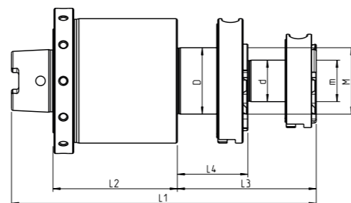
Walter HSK40A: gestufter Schaft
