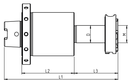
Walter HSK40A: standard-Schaft
